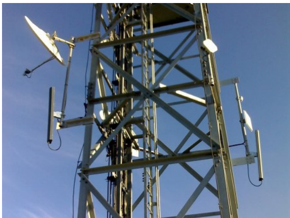
Abbildung 6: Parabolantennen für Richtfunk, die anderen verteilen an umliegende Häuser.
